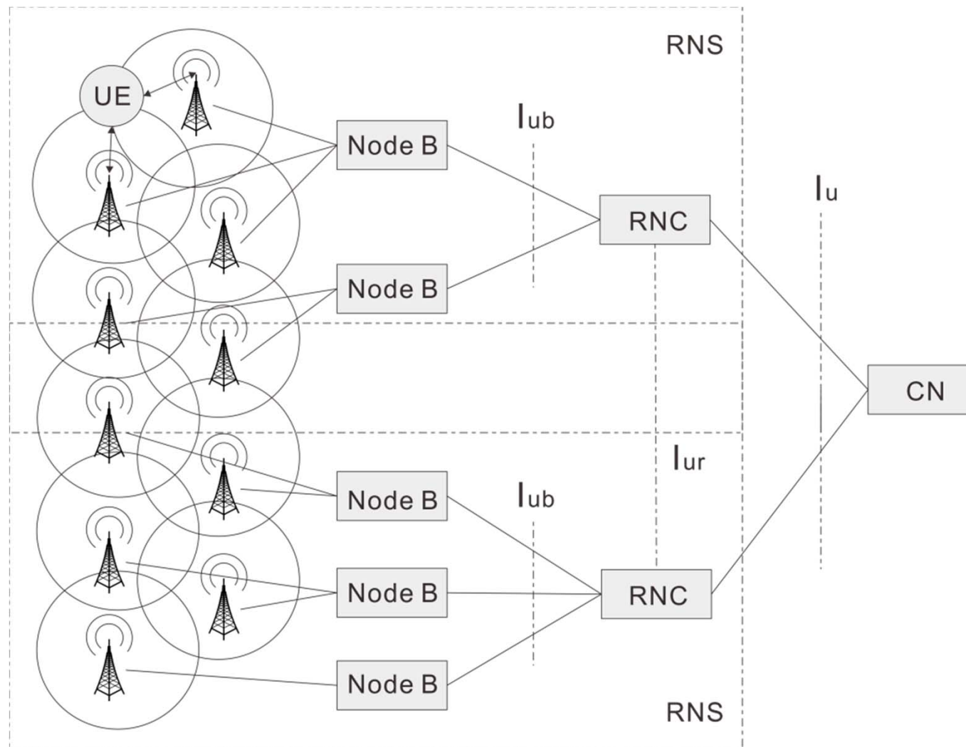
圖9: UTRAN架構
