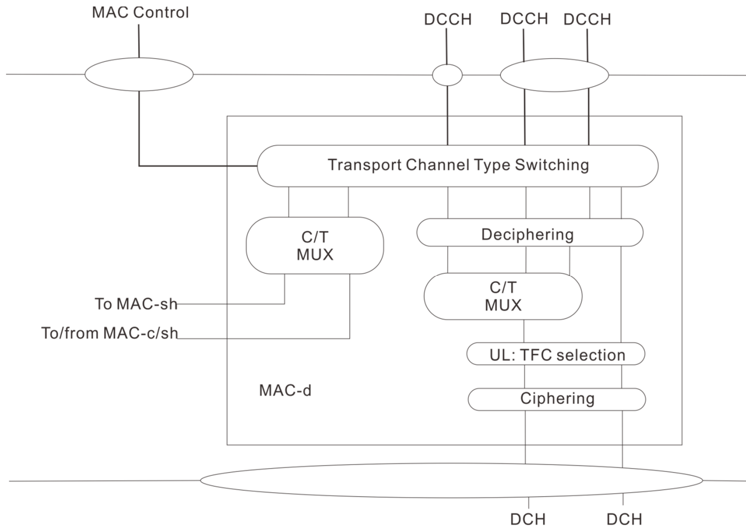
圖 15: UTRAN端MAC-d層架構圖
